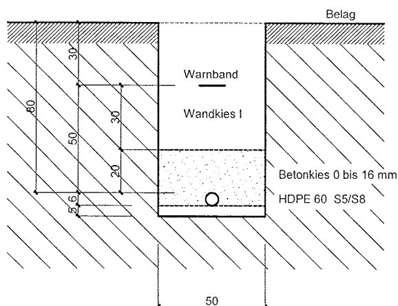
Profil Strasse
