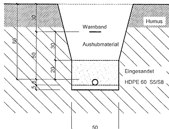
Profil Wiese
